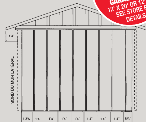
No 3 MUR ARRIÈRE EN 2 x 4
